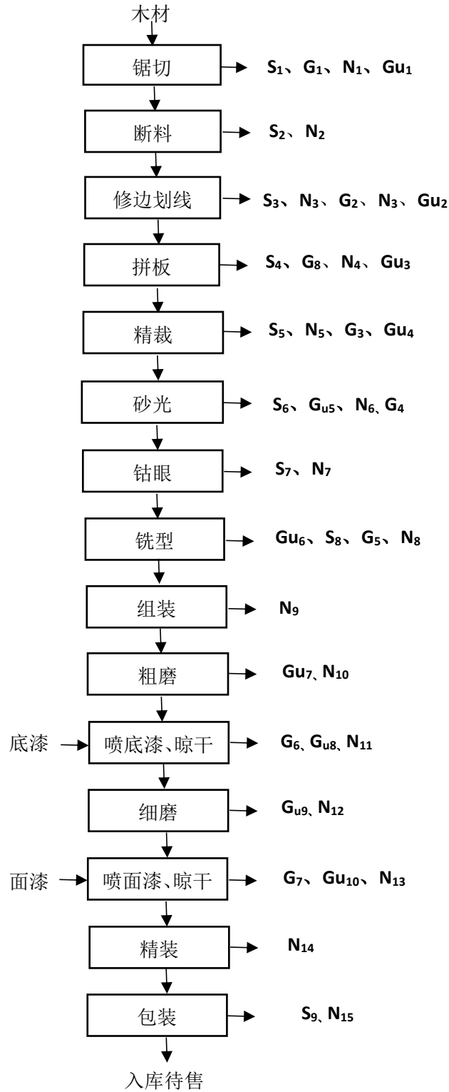
图 2 生产流程图
